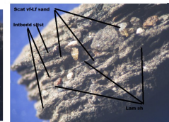
Montney Turbidite
